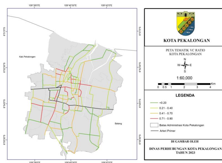
Gambar II-47 Peta V/C Ratio Ruas Jalan di Kota Pekalongan
